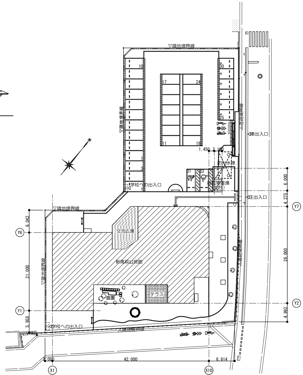
配置図
