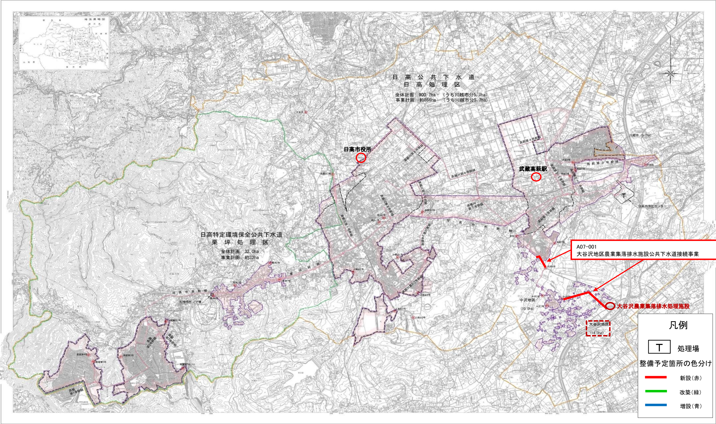
日高公共下水道汚水計画一般図
