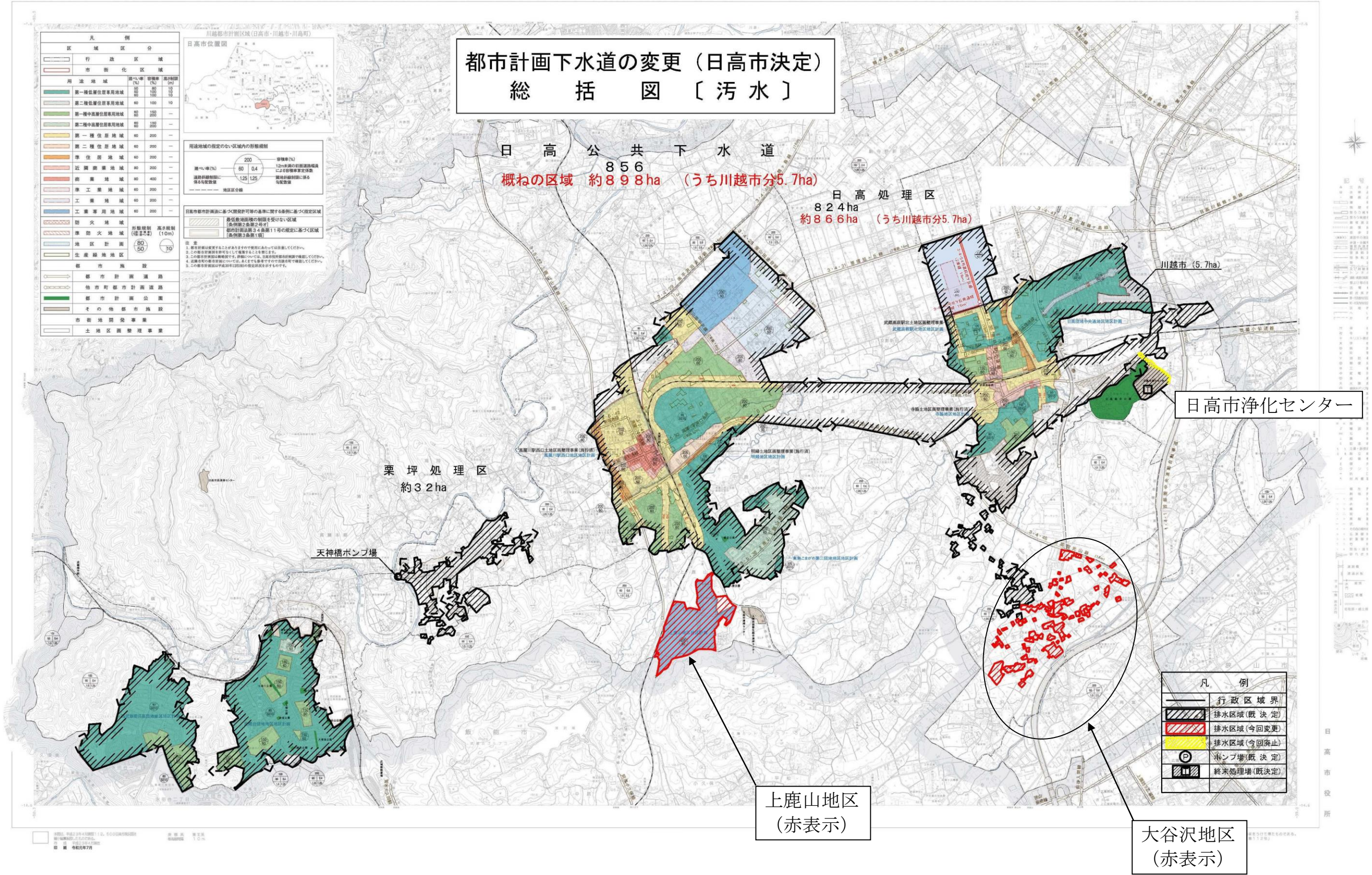
図－1 総括図（汚水）
