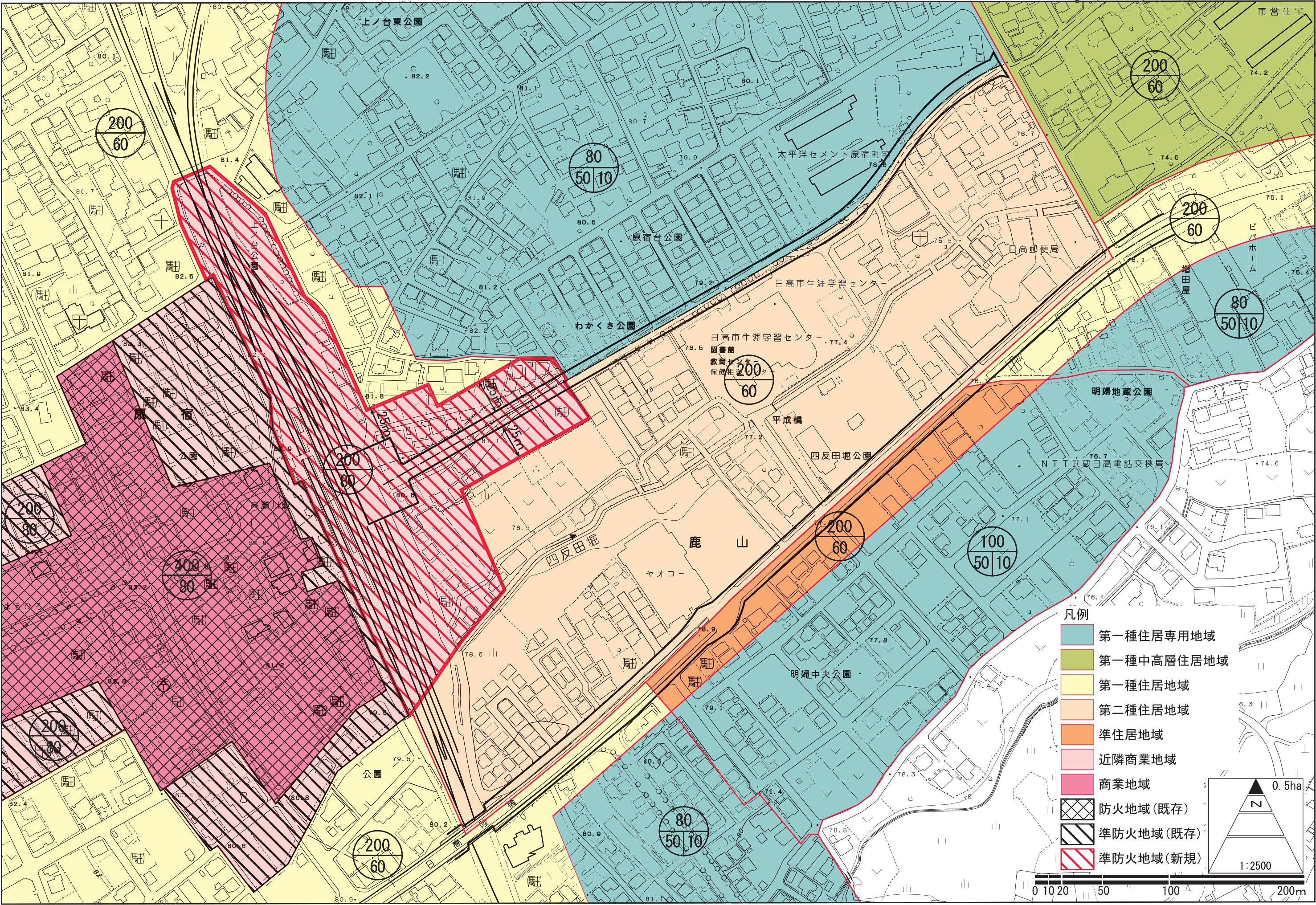
計画図（防火地域及び準防火地域）（変更後）
