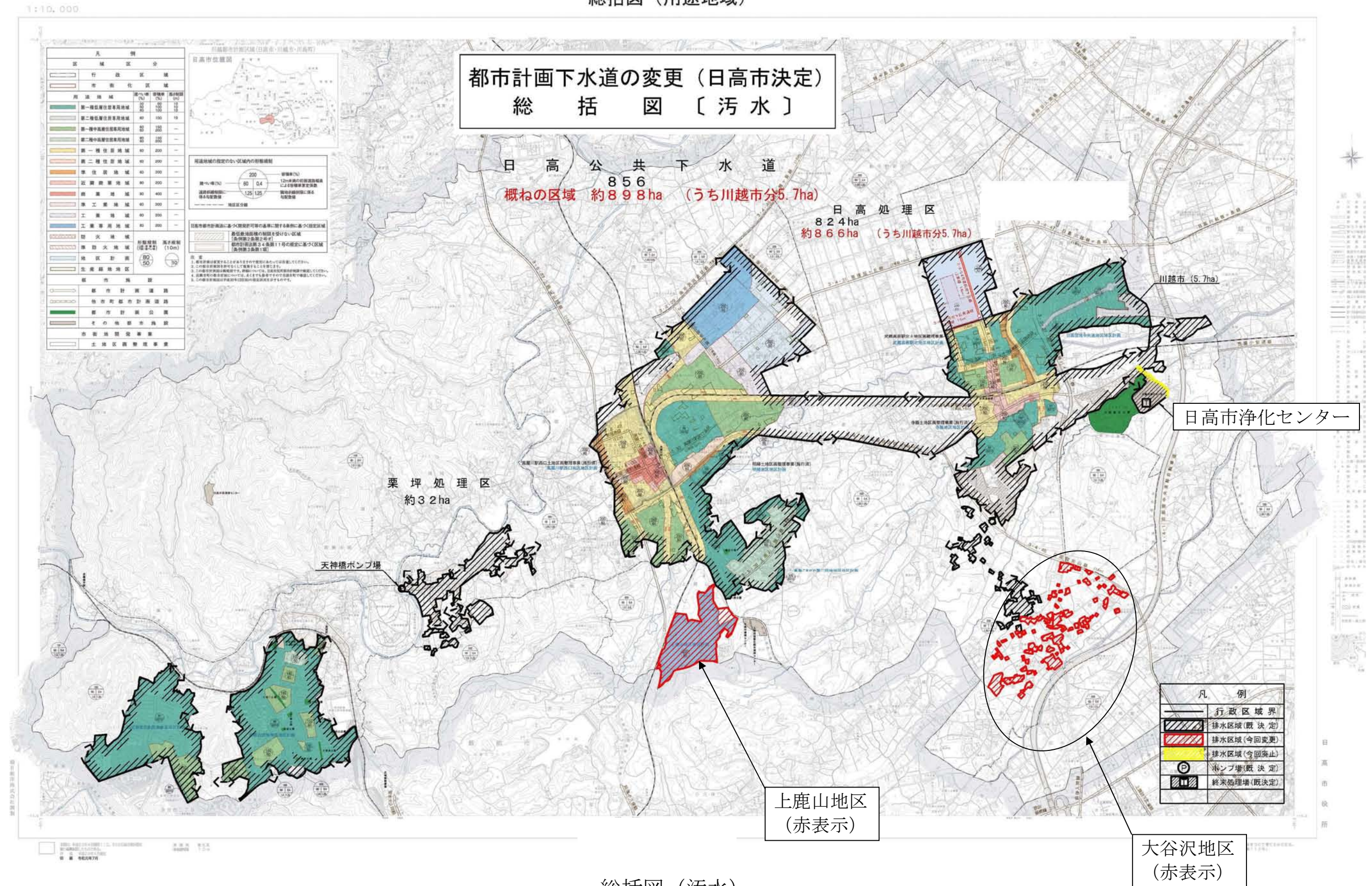
総括図（汚水）
