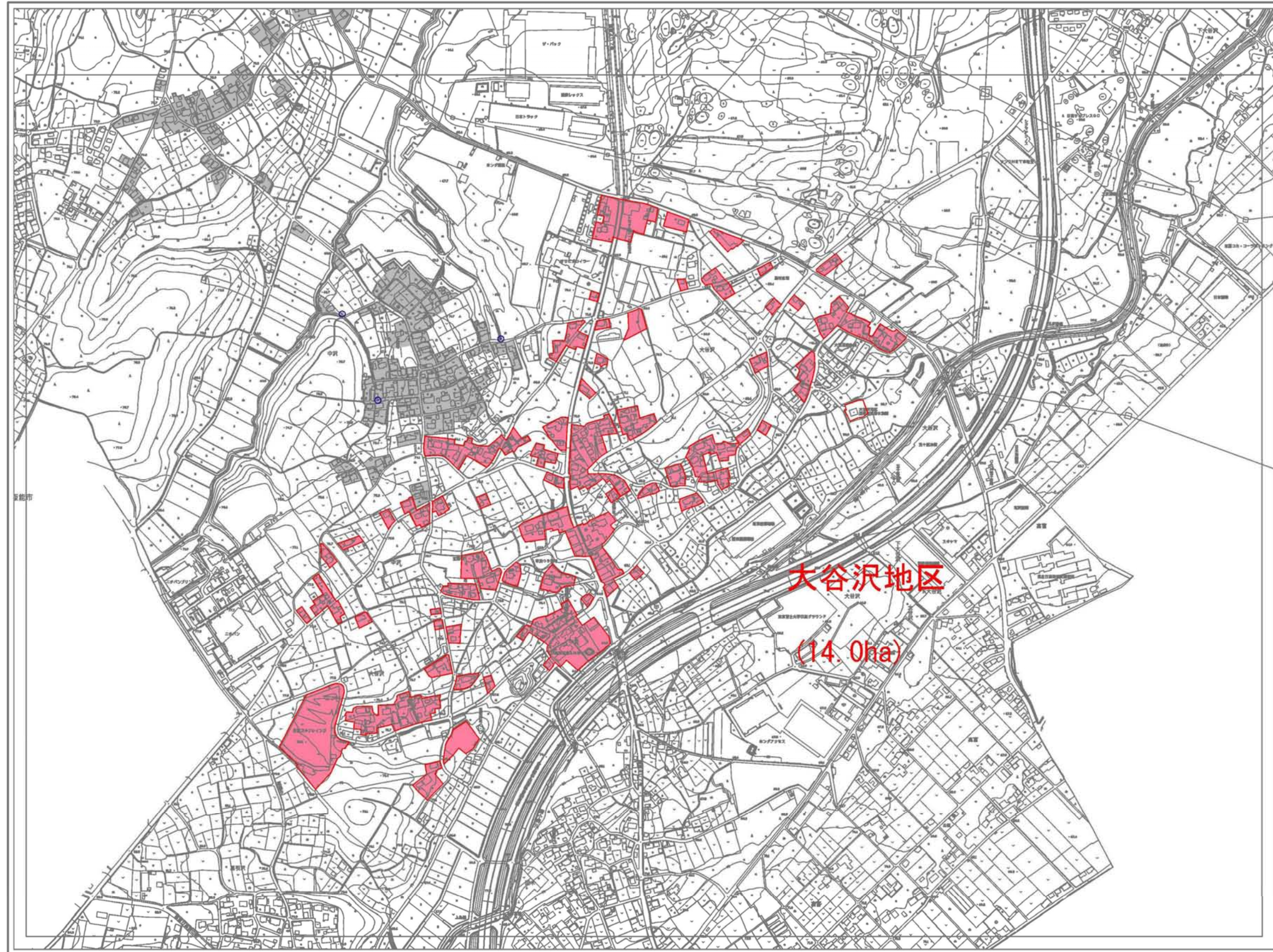
計画図 (大谷沢地区)
