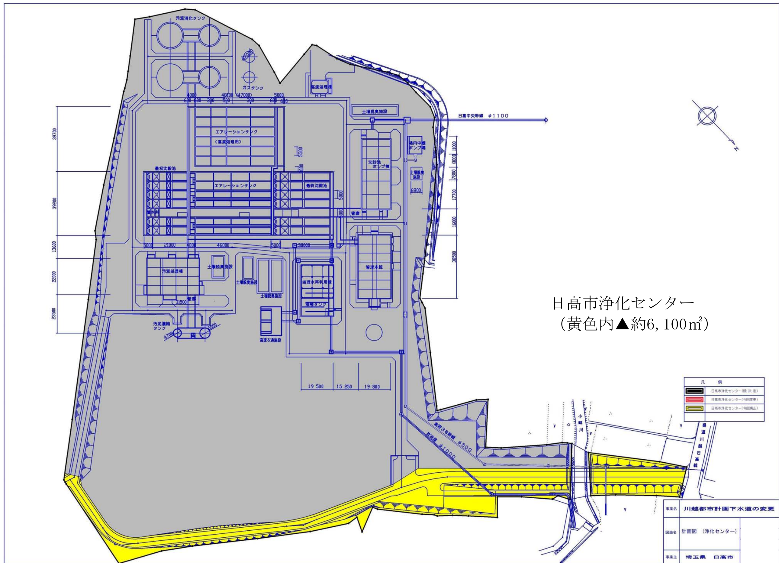
計画図 (日高市浄化センター)
