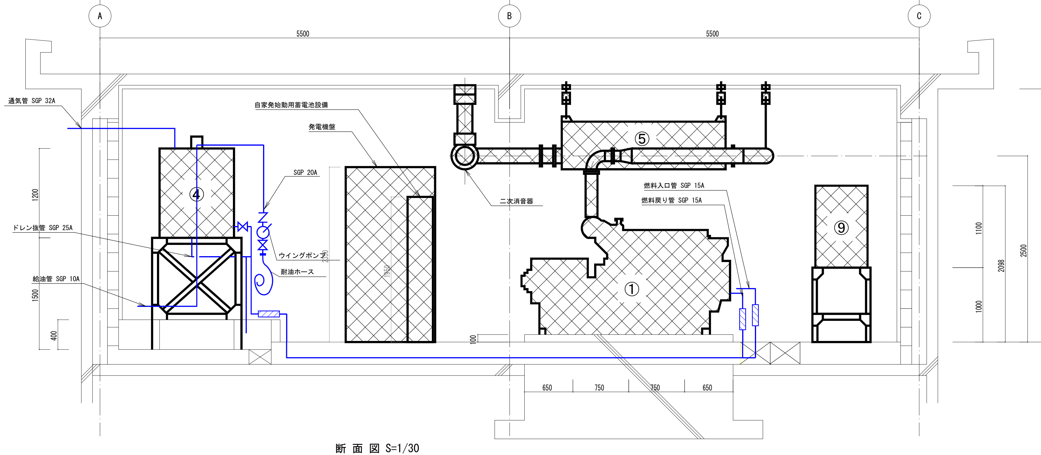
断面図 S=1/30
