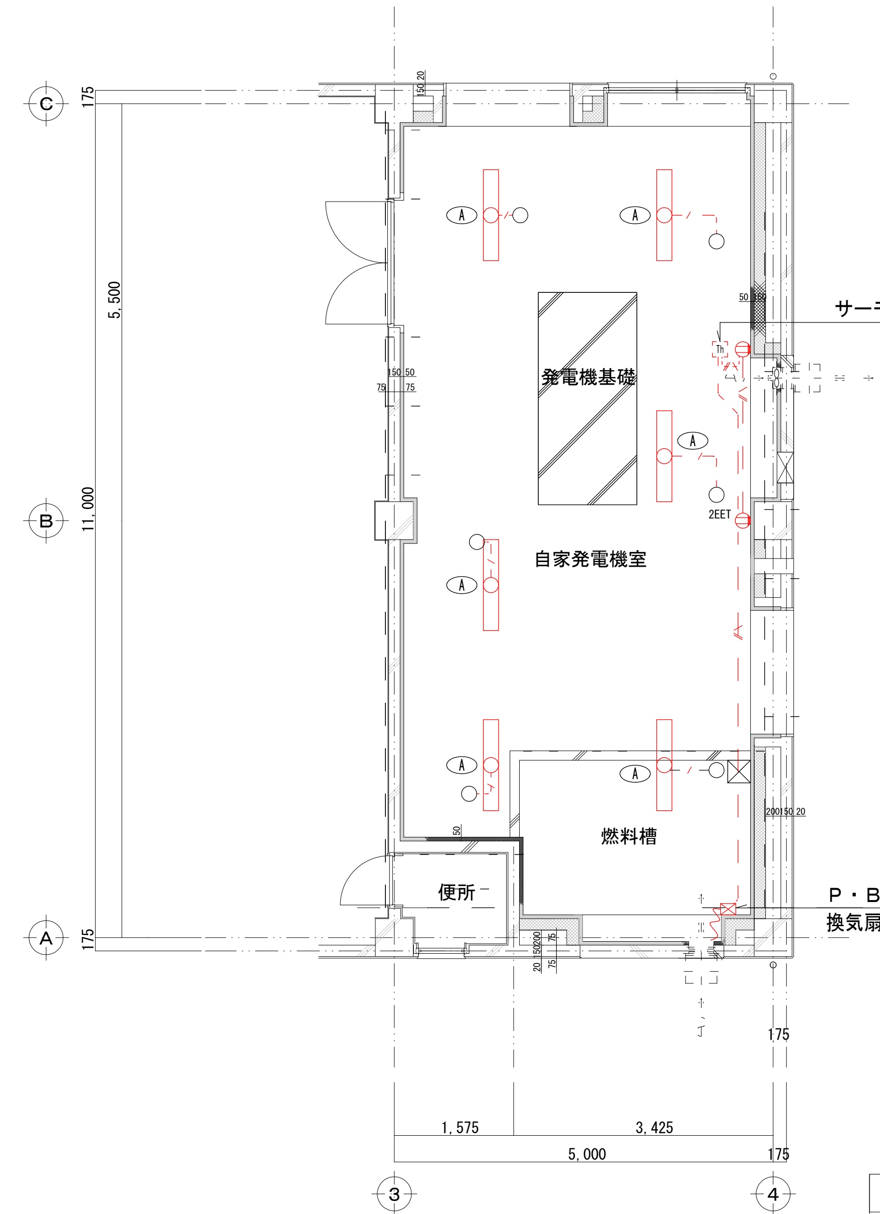
改修後 電気設備平面図 S=1/50
