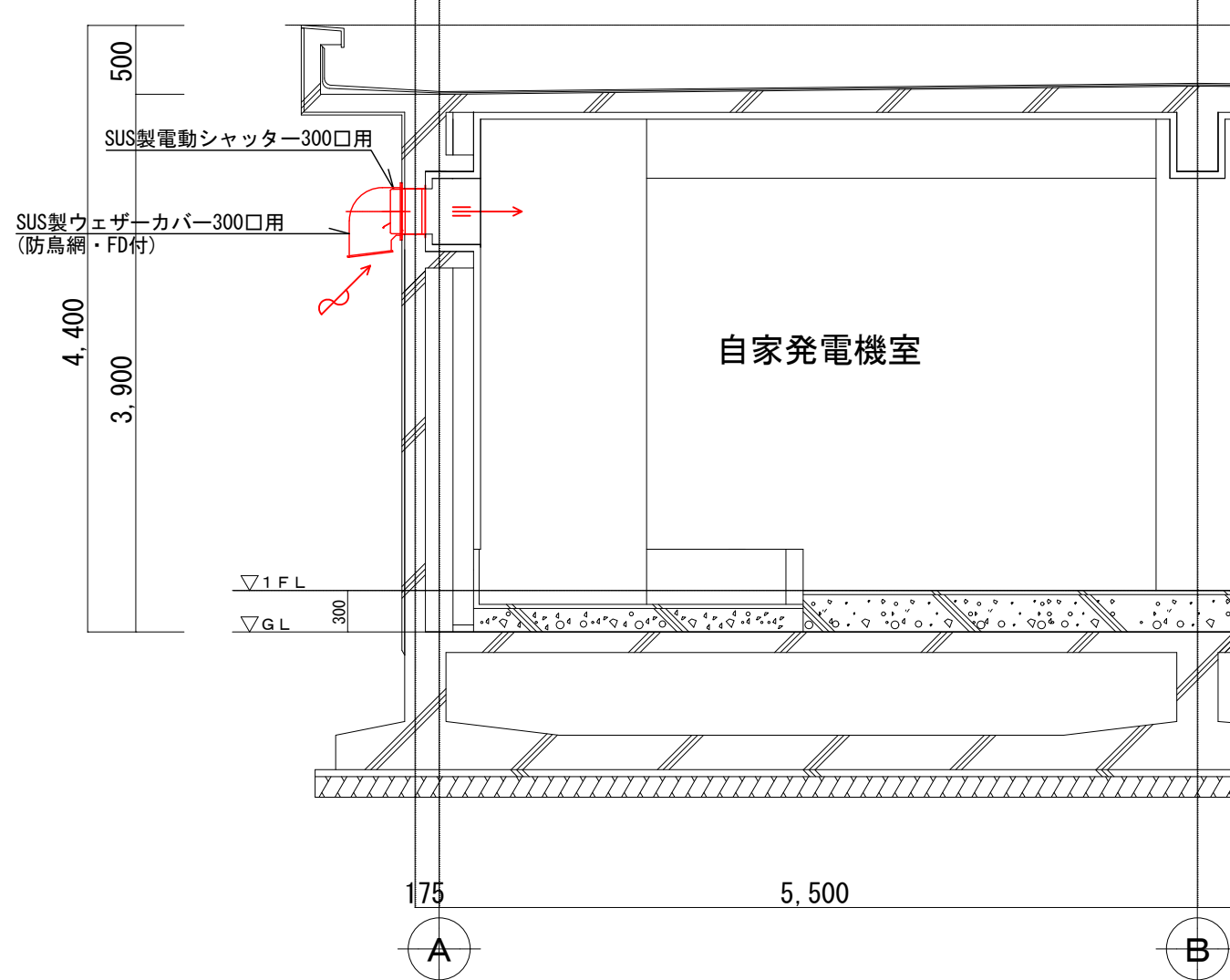
口一口改修後断面図 S=1/50
