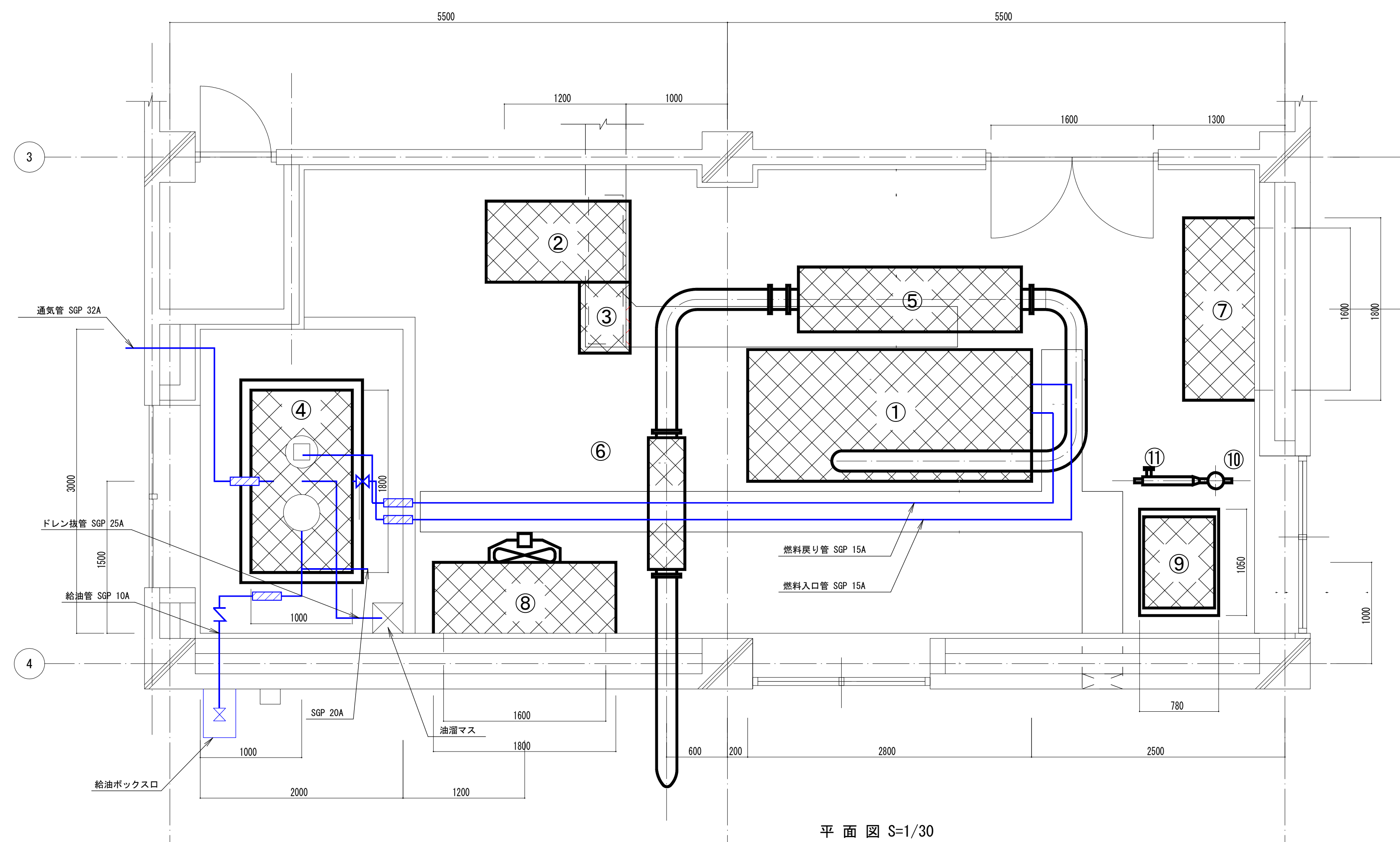
平面图 S=1/30
