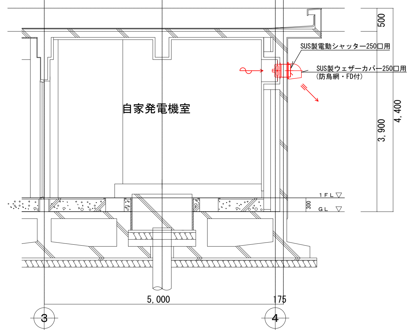
イーイ改修後断面図 S=1/50
