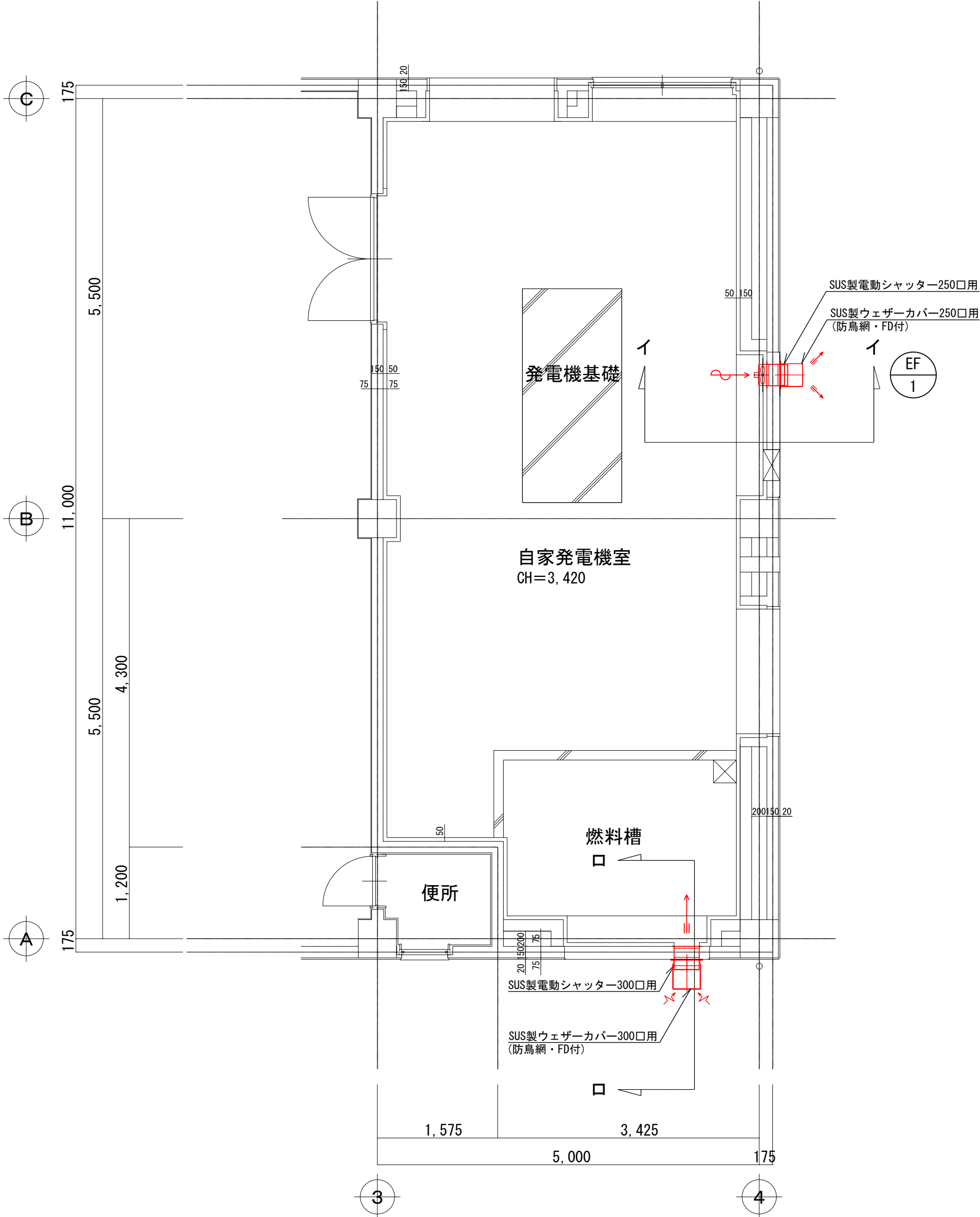
改修後 換氣設備平面図 S=1/50
