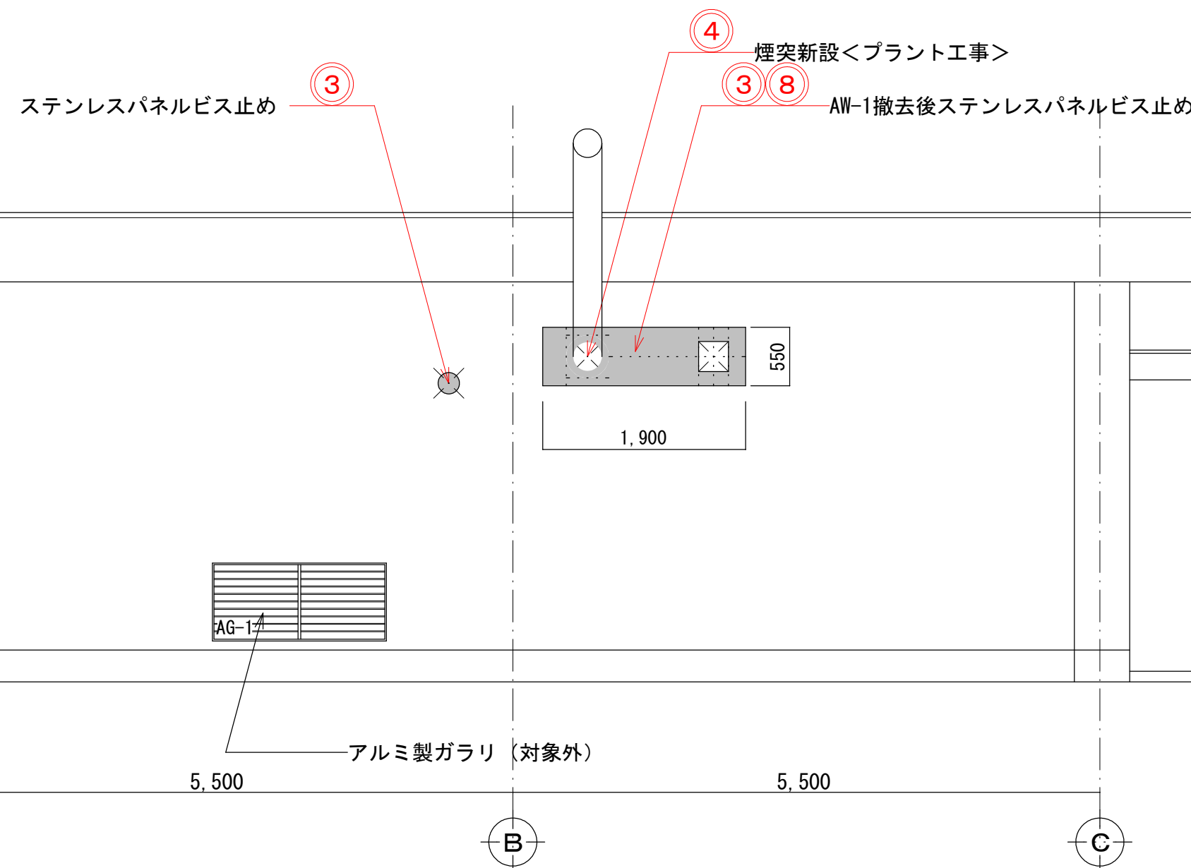
改修後 東側立面図 S=1/50
